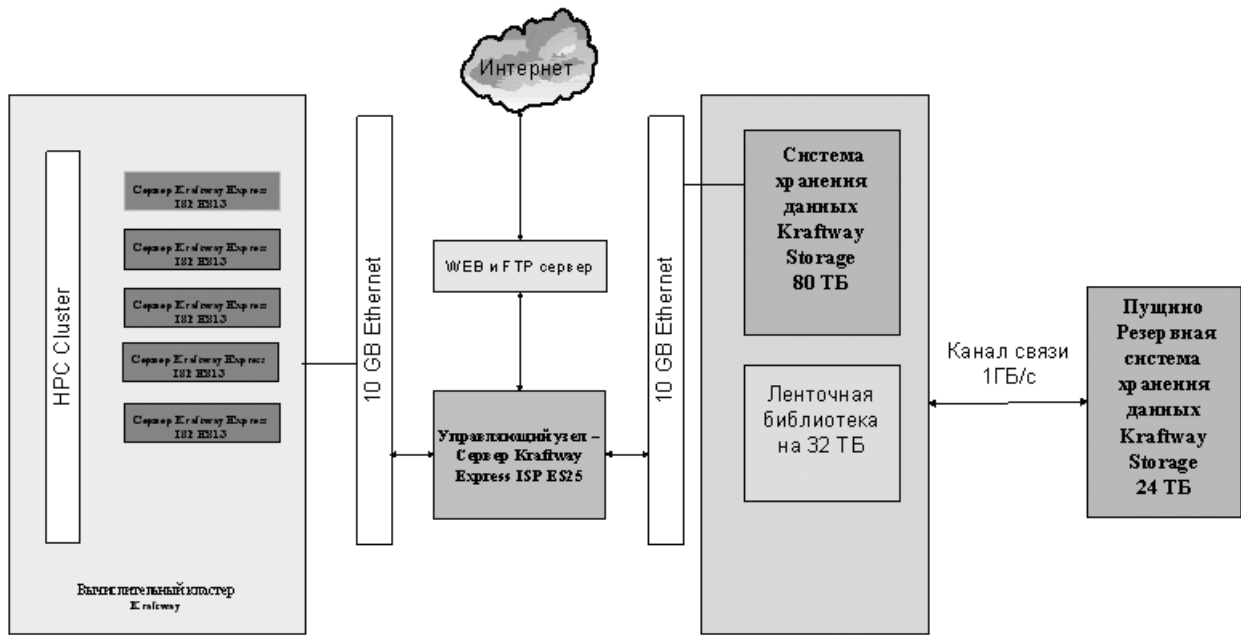
Рис. 1. Архитектура вычислительного комплекса
