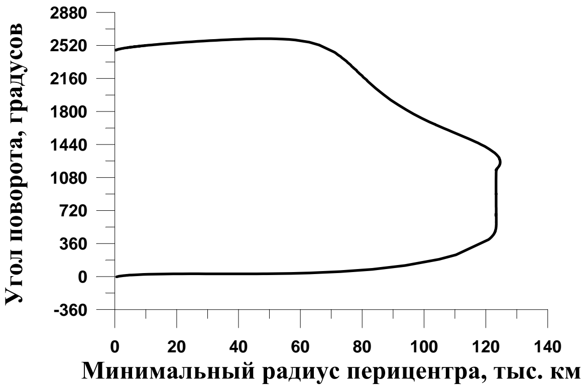
Рис 13. Семейство орбит соизмеримости 5/2\nu
