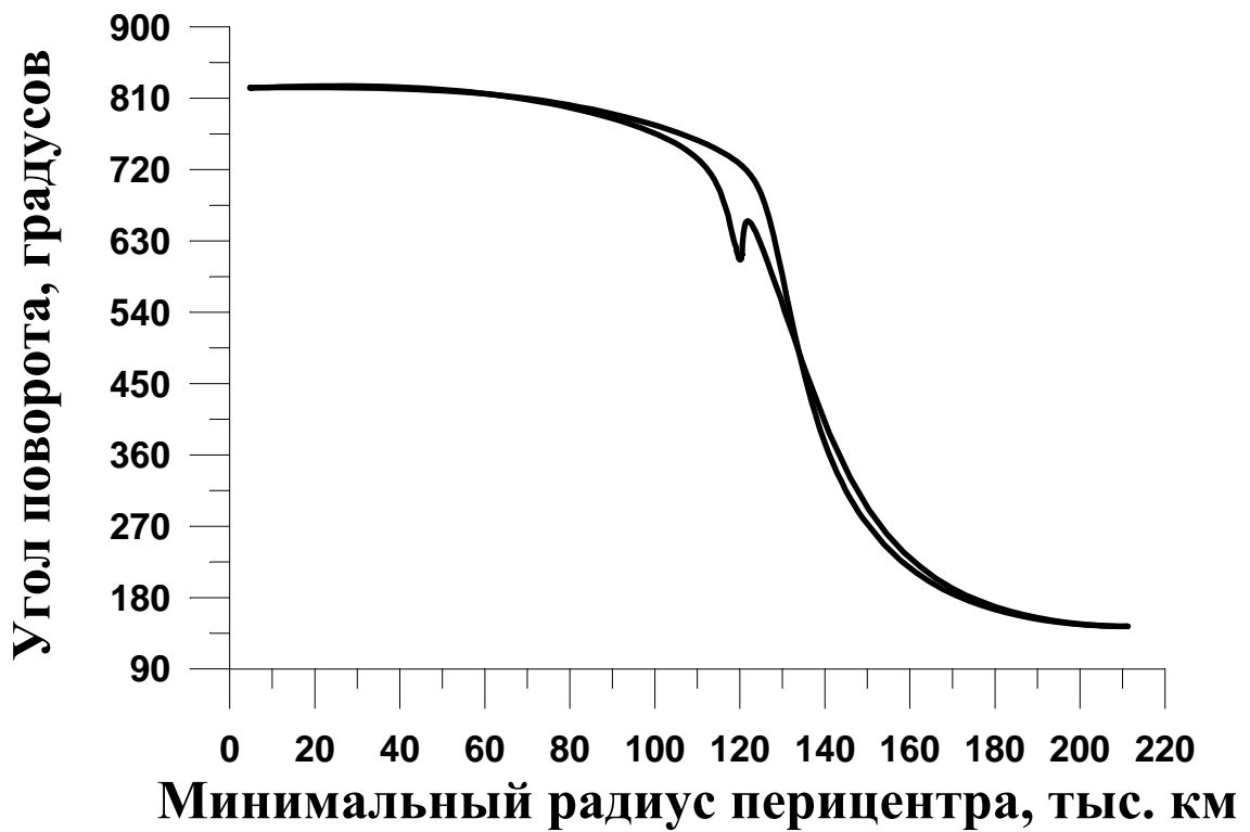
Рис 10. Семейство орбит соизмеримости 11/5
