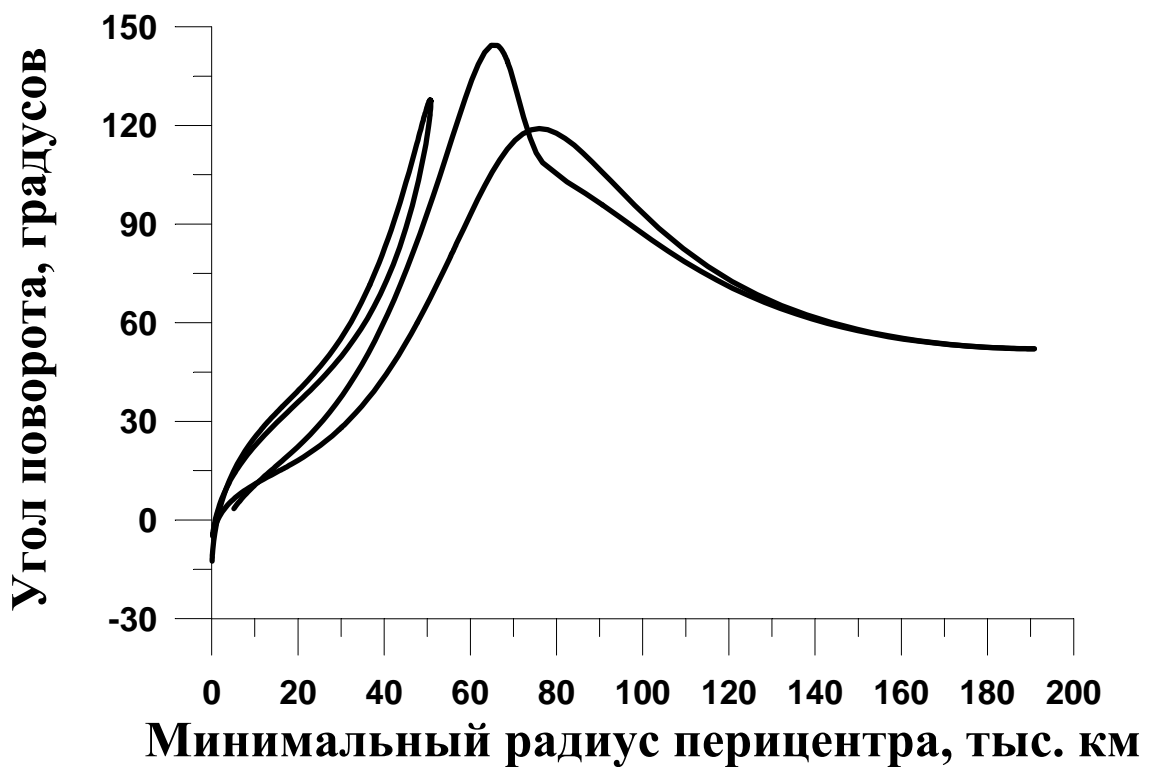
Рис 2. Семейство орбит соизмеримости 14/5
