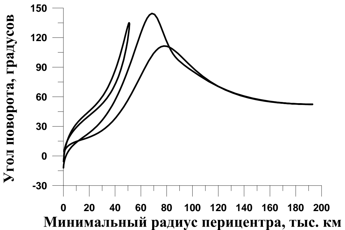
Рис 3. Семейство орбит соизмеримости 11/4
