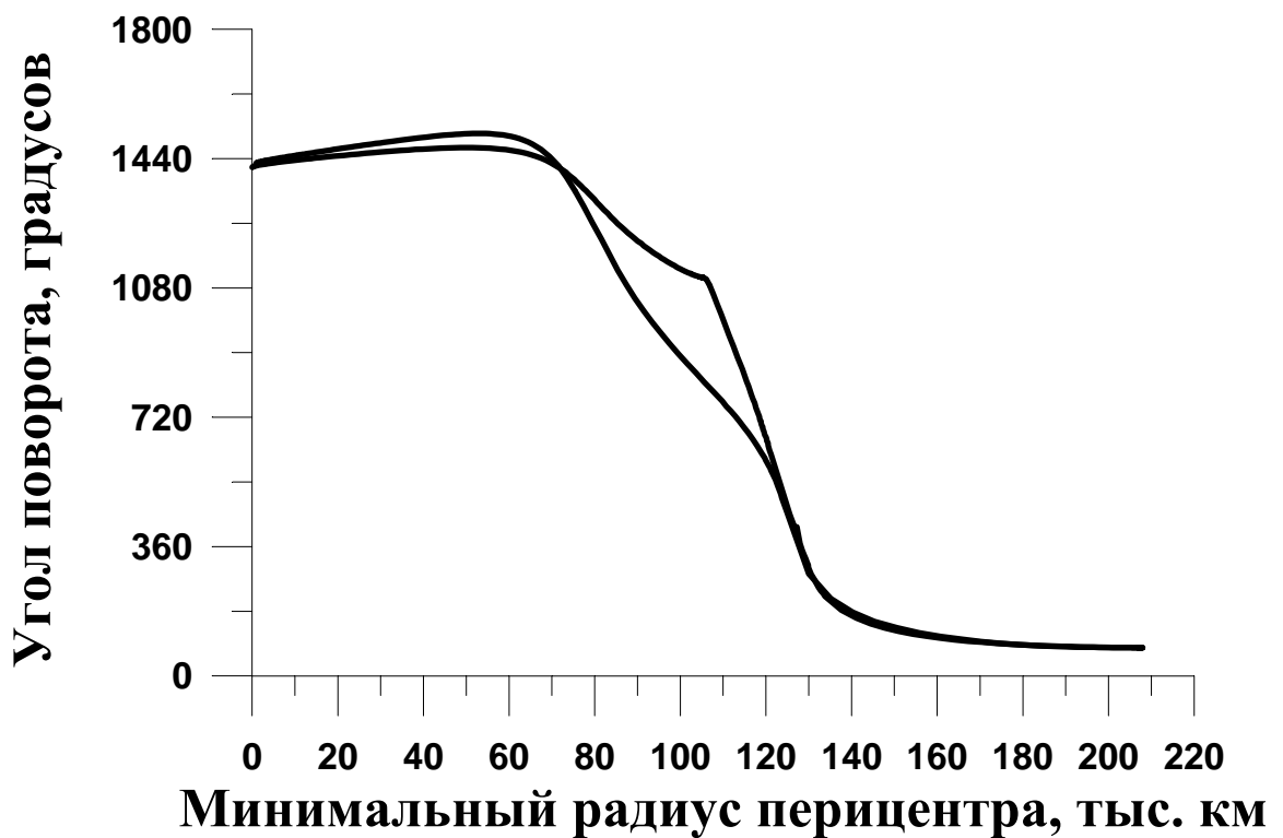
Рис 7. Семейство орбит соизмеримости 12/5
