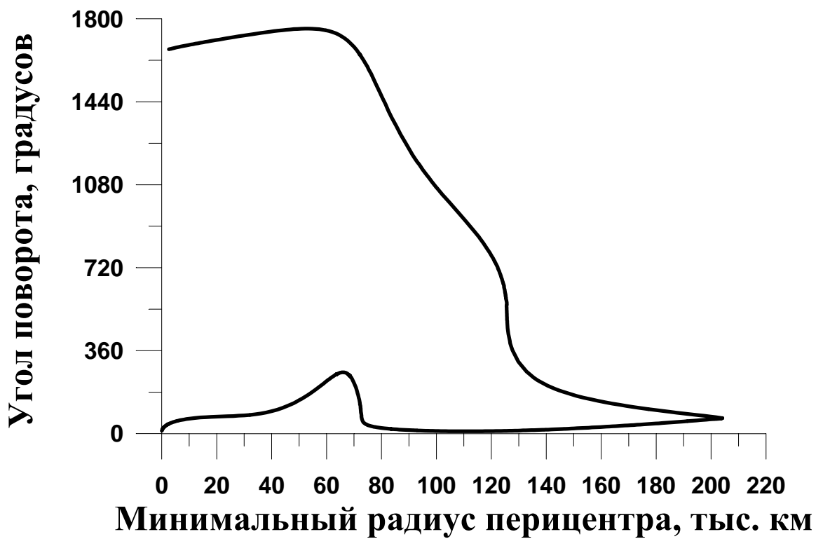
Рис 6. Семейство орбит соизмеримости 5/2
