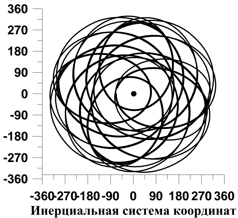
Рис. 16. Орбита семейства 7/3\nu
