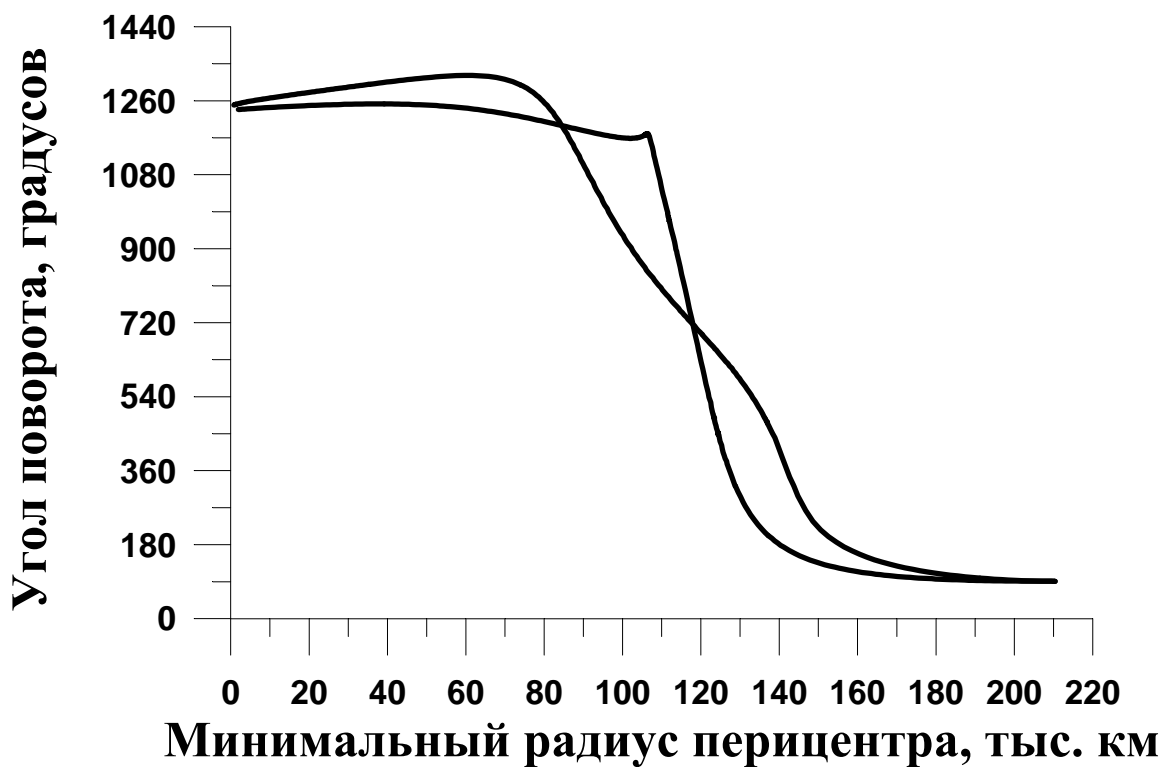
Рис 8. Семейство орбит соизмеримости 7/3n
