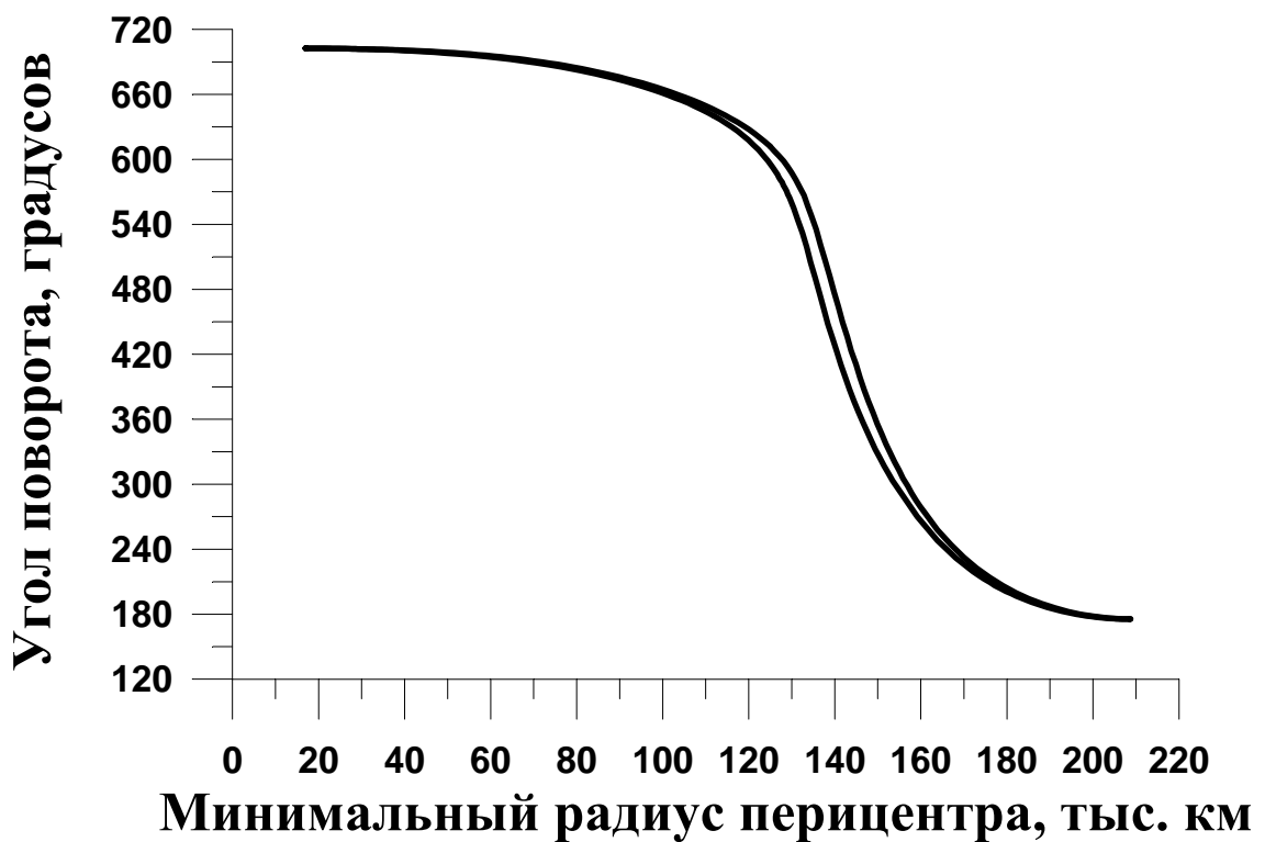
Рис 11. Семейство орбит соизмеримости 13/6
