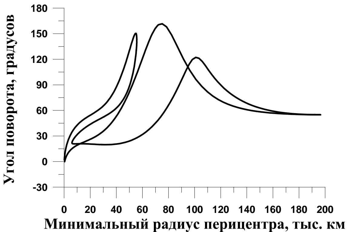
Рис 4. Семейство орбит соизмеримости 8/3n
