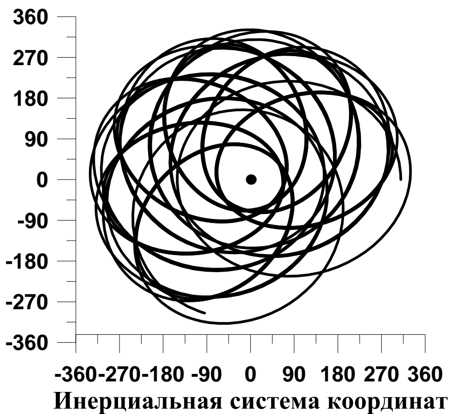
Рис. 15. Орбита семейства 5/2\nu
