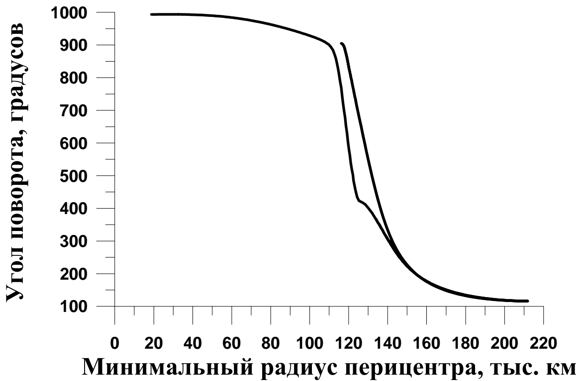
Рис 9. Семейство орбит соизмеримости 9/4
