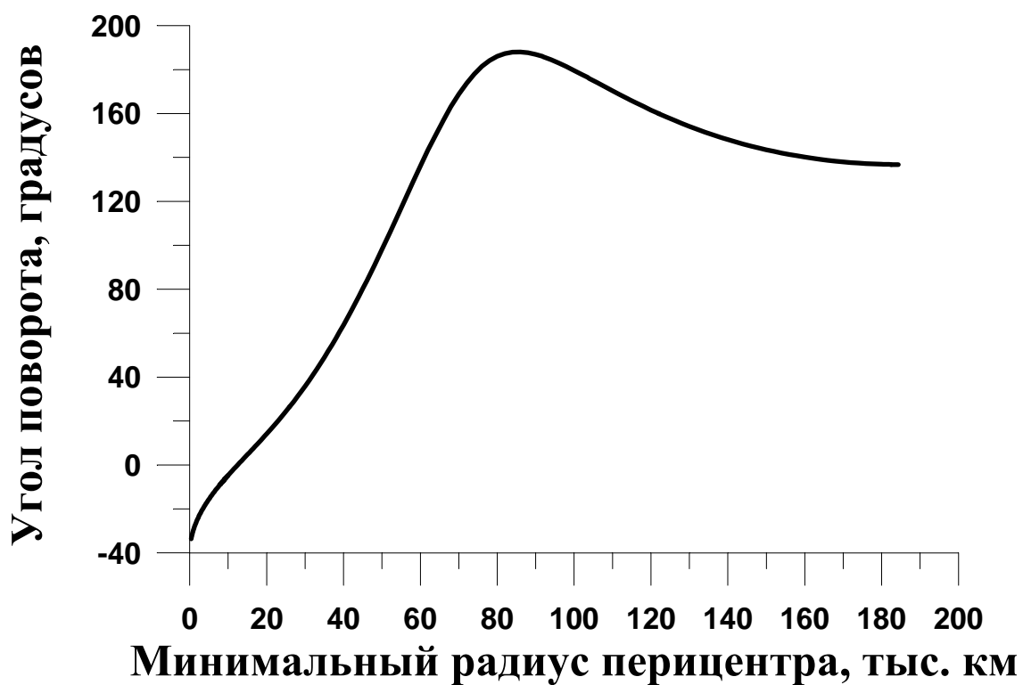
Рис 1. Семейство орбит соизмеримости 3/1
