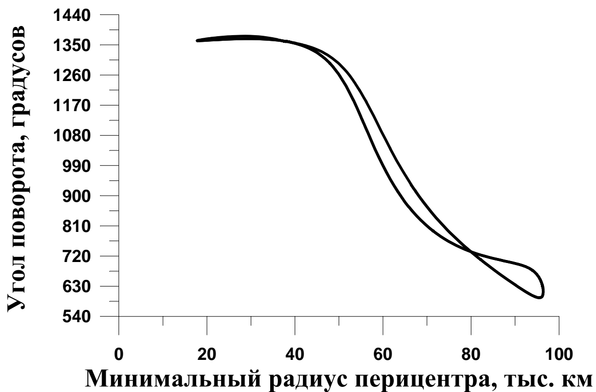
Рис 12. Семейство орбит соизмеримости 8/3\nu
