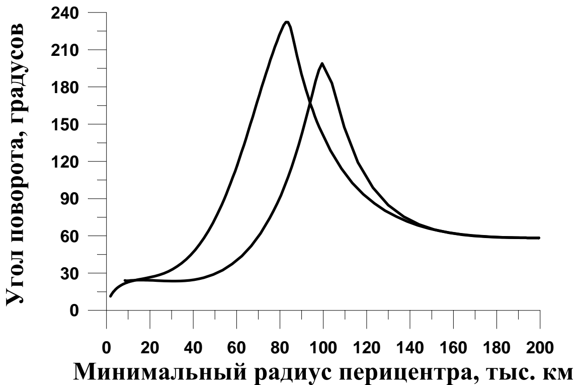
Рис 5. Семейство орбит соизмеримости 13/5
